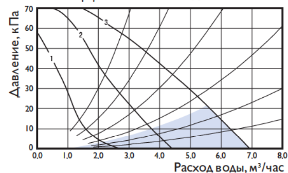
ВДЛ-300А-83-12 ВДЛ-300Т-83-12
