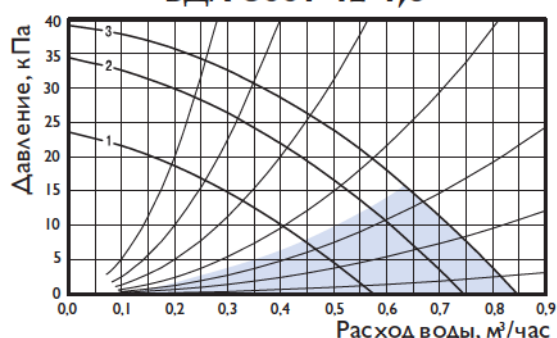
ВДЛ-300А-42-1,6 ВДЛ-300Т-42-1,6
