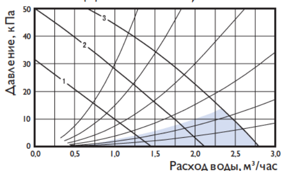
ВДЛ-300А-62-6,3 ВДЛ-300Т-62-6,3
