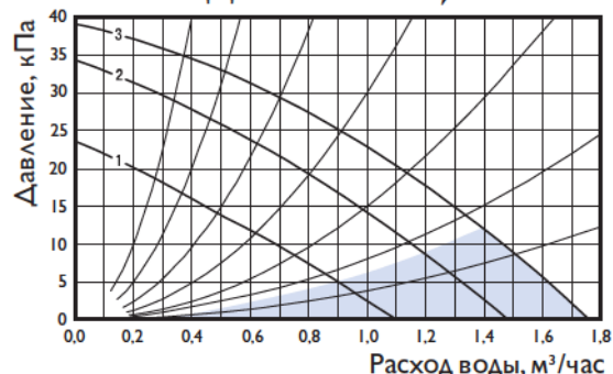
ВДЛ-300А-42-4,0 ВДЛ-300Т-42-4,0
