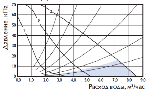
ВДЛ-300А-83-15 ВДЛ-300Т-83-15
